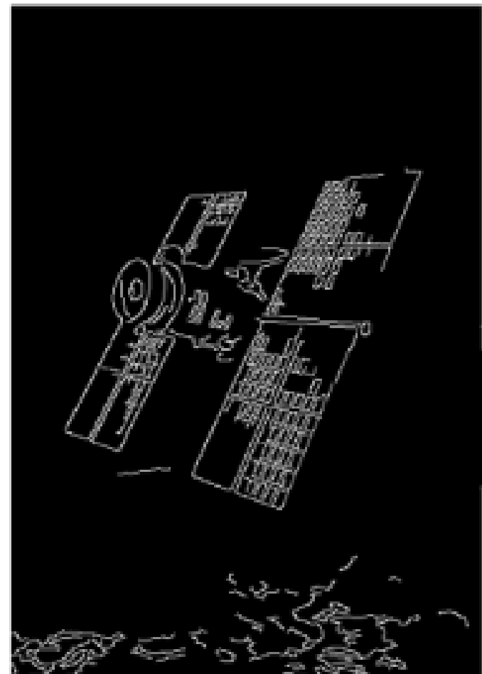
Edge Detection
